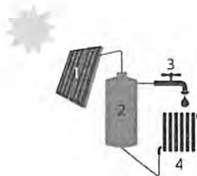
1 Zonnecollector | 2 Opslagvat zonnewater 3 Sanitair warmwater 4 Ruimteverwarming Wolven
