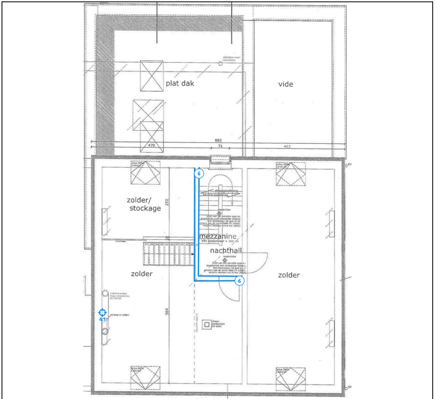
Legende van plan 1.3: Hoofdgebouw plan - pleister muren
