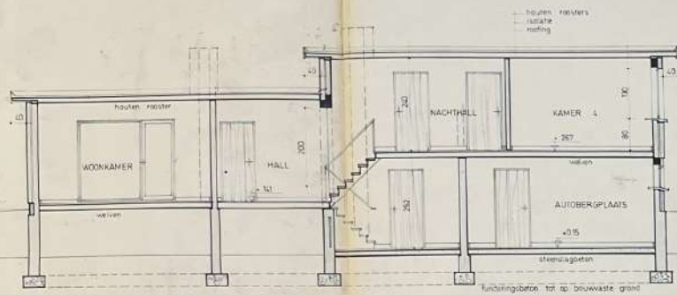
LENGTEDOORSNEDE : C-D
