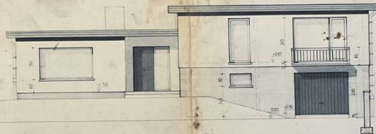
STRAATGEVEL
