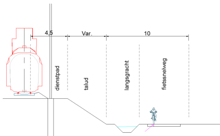
Figuur 1 Schematische voorstelling van de bouwvrije strook
