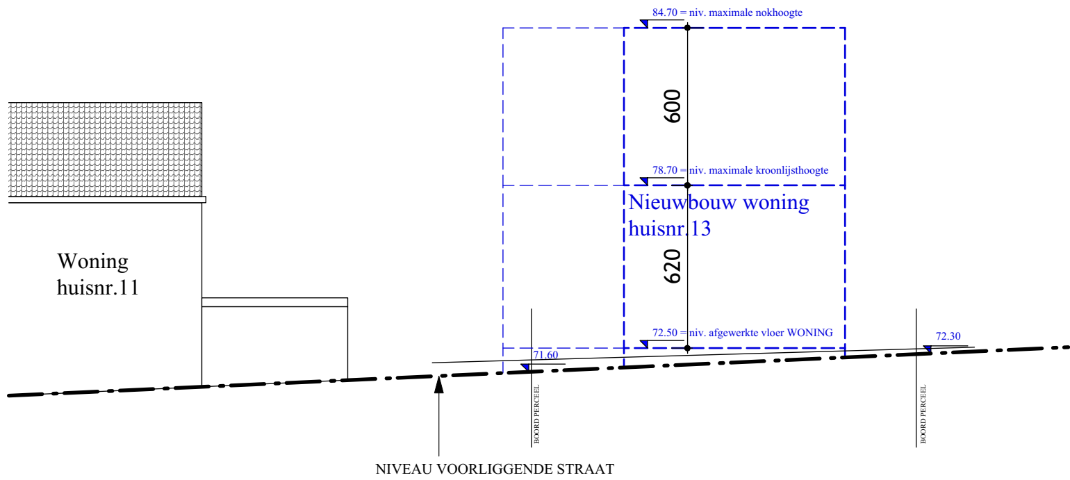
TERREINPROFIEL 1 SCH 1/200
