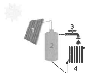
Zonnecollectoren zetten de energie van de zon om in warmte. Een zonneboilerinstallatie bestaat uit zonnecollectoren op het dak en een opslagvat voor warm water. Een zonneboiler verwarmt een deel van het sanitair warm water met gratis zonnewarmte. Als de installatie voldoende groot is, kan ze ook in een deel van uw behoefte voor ruimteverwarming voorzien. Hou er wel rekening mee dat een zonnecollector het hoogste rendement behaalt in de zomer. Het rendement in de winter ligt beduidend lager.
