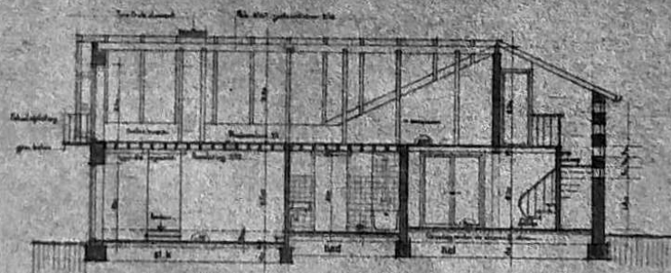
DOORSNEDEN EF
