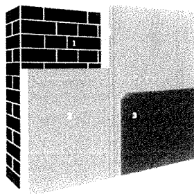
1. Buitengevel | 2. Isolatie | 3. Dampschermb | 4. Binnenafwerking | 5. Stijl- en regelwerk (optioneel)
