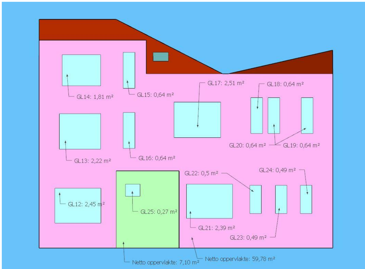
FIGUUR 3: ACHTERGEVEL
