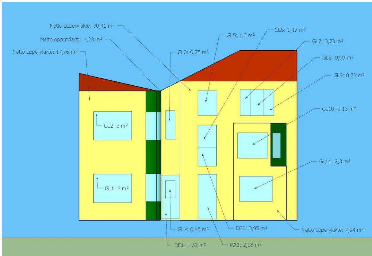
FIGUUR 2: VOORGEVEL
