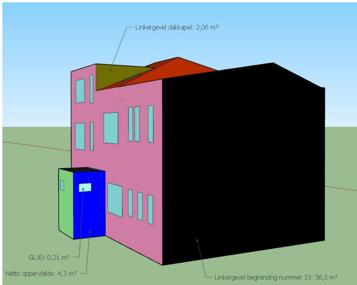
FIGUUR 5: LINKERGEVEL
