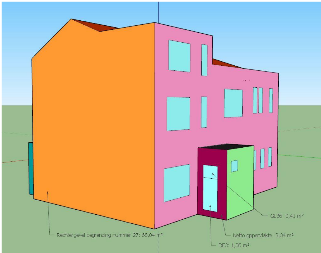
FIGUUR 7: RECHTERGEVEL
