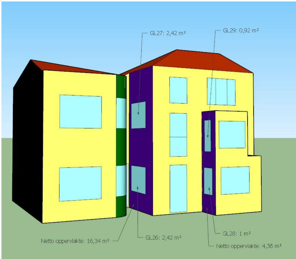
FIGUUR 4: LINKERGEVEL
