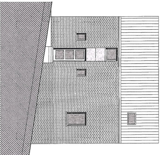
FACADE AVANT
