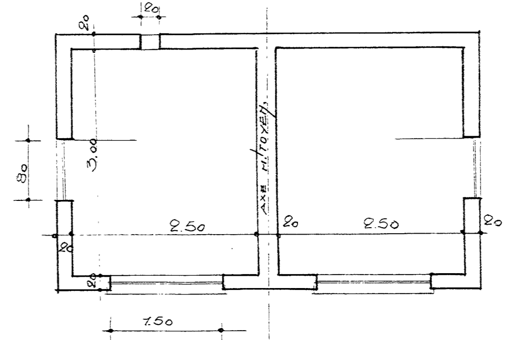
LOCAL D'ELEVAGE.
