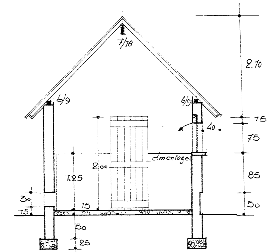
LOCAL D'ELEVAGE.
