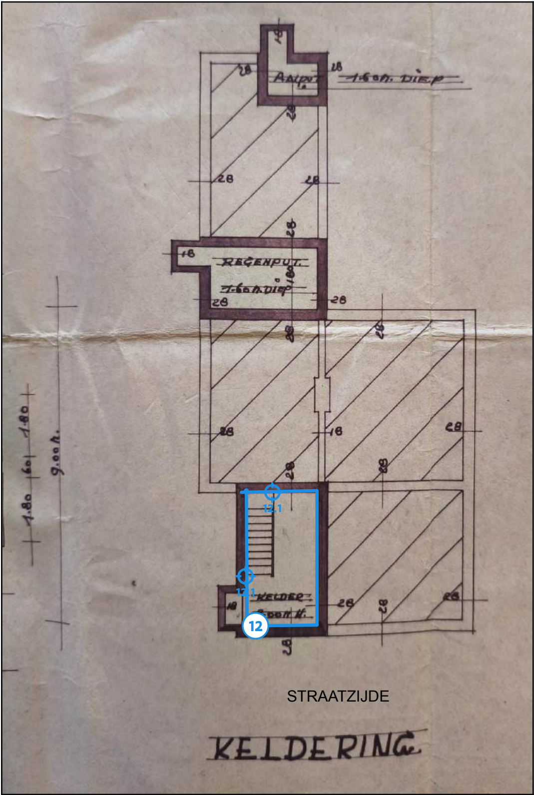
Legende van plan 1.1: Kelder
