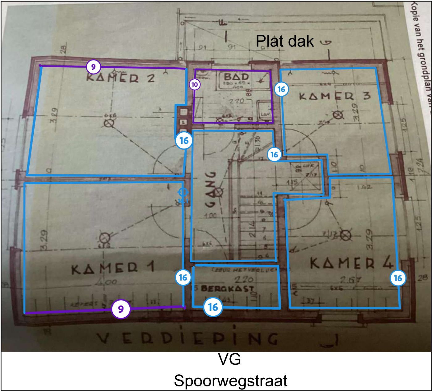
Legende van plan 1.5: 1ste verdieping
