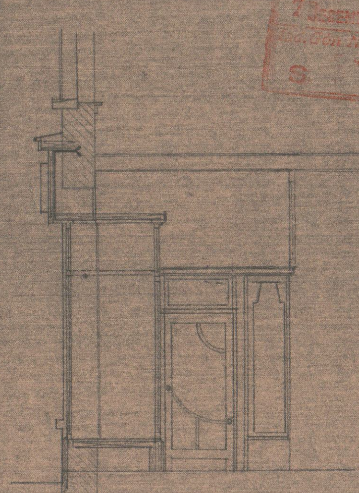
DOORSNEDEN C-D
