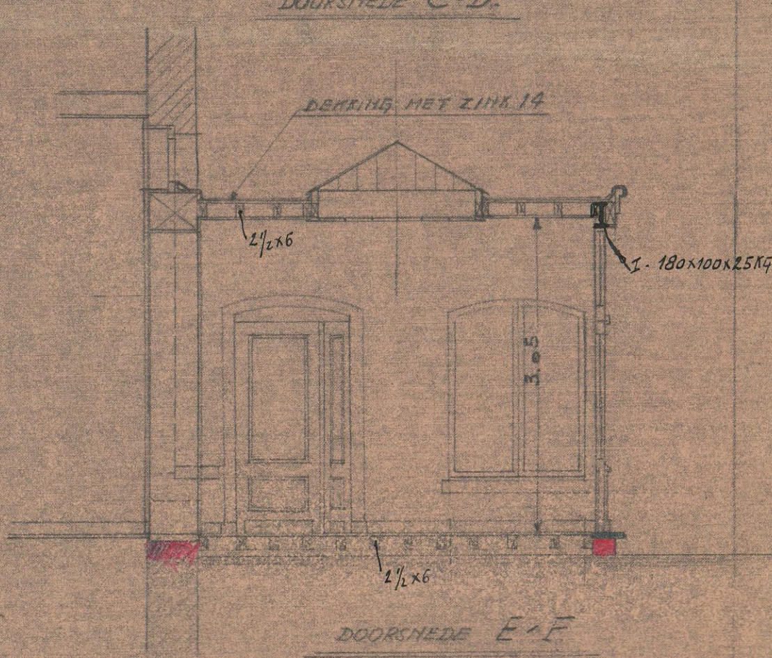
DOORSNEDEN E-F
