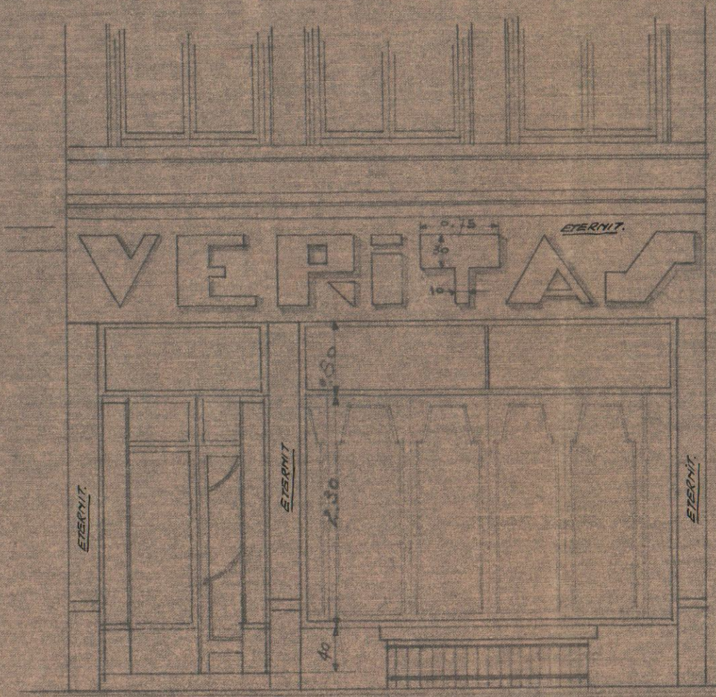
GEWIJZIGDE VOORGEVEL
