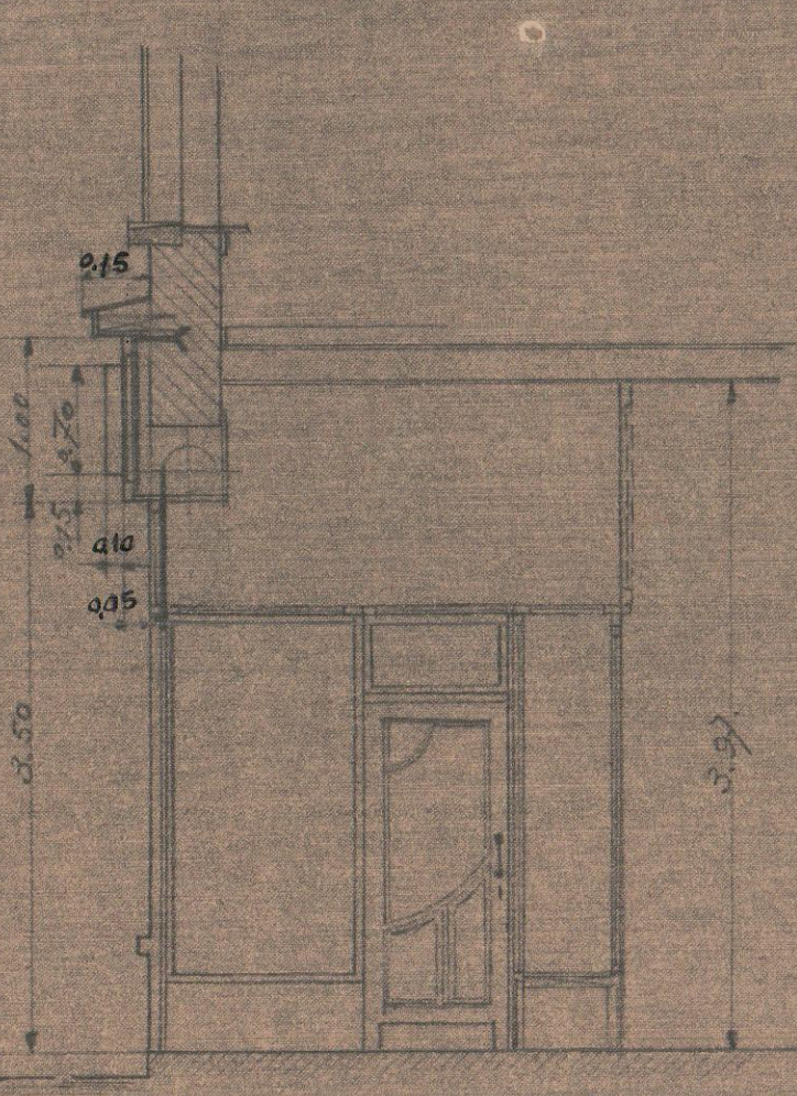
DOORSNEDEN A-B
