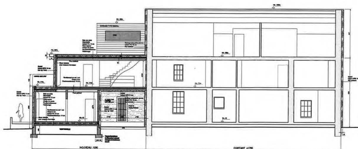
COUPE BB
